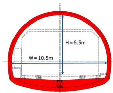
標準断面図
